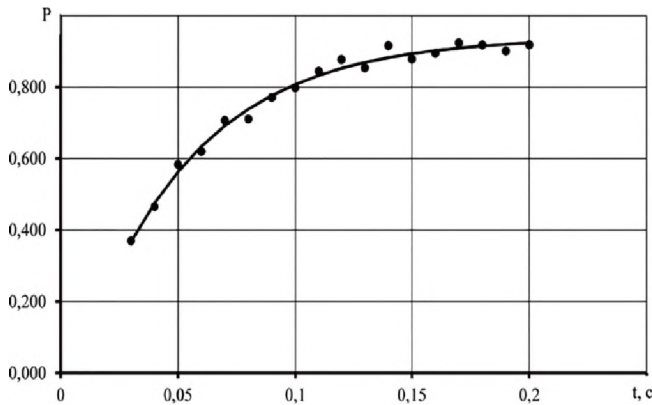
Рисунок 3 – Залежність ймовірності реагування газової форсунки P на інтервал часу t між двома насінинами, які падають
