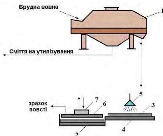
Рис. 1. Техніко-технологічний модуль ТТМ-1П
