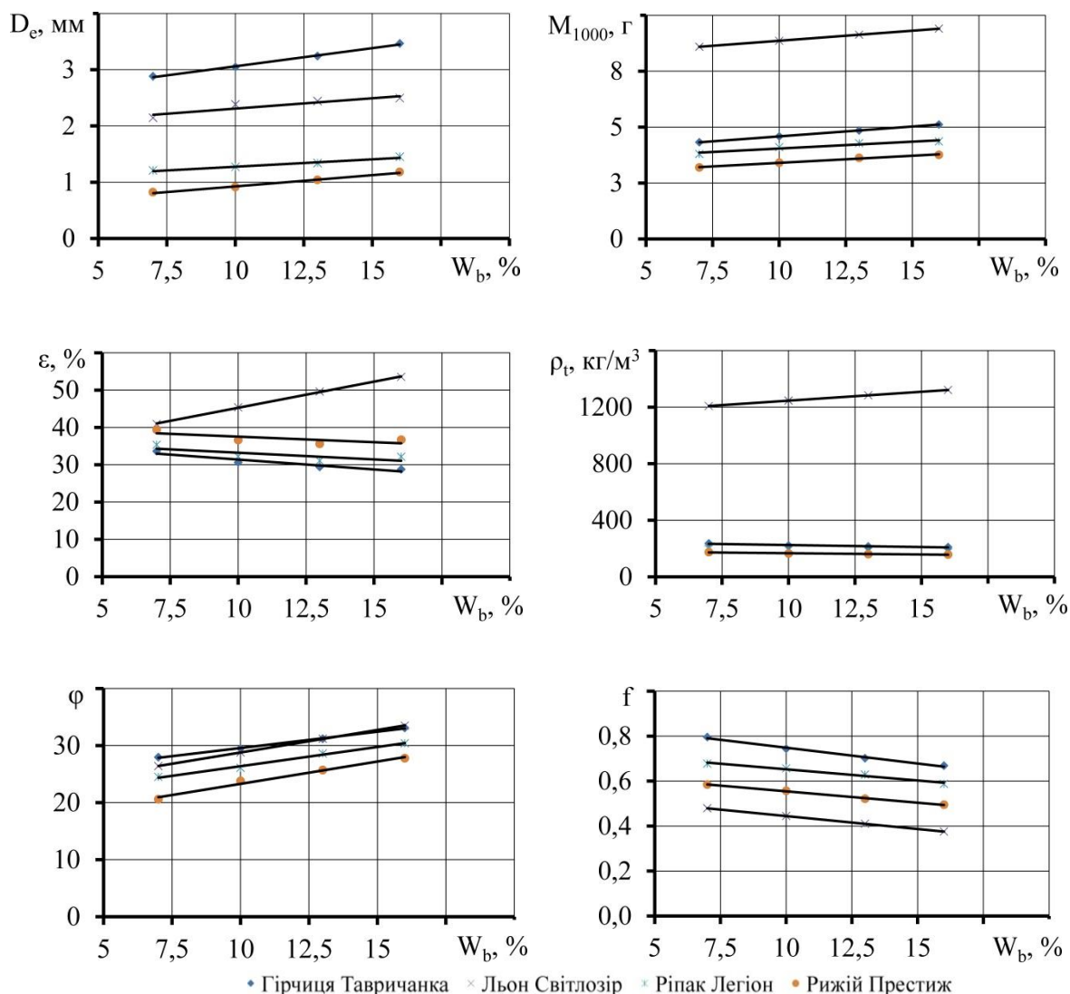
Рисунок 3 – Залежність впливу вологості насіння W_b на ефективний діаметр D_e , масу 1000 насінин M_{1000} , пористість \varepsilon , дійсну щільність \rho_t , кут природного ухилу \varphi , коефіцієнт тертя f Джерело: розроблено авторами
