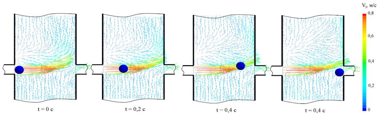
Рис. 1. Процес переміщення насінини з об'єму забірної камери в насіннепровід: n = 0,32 , \alpha = 15^\circ , V_0 = 0,6 м/с
