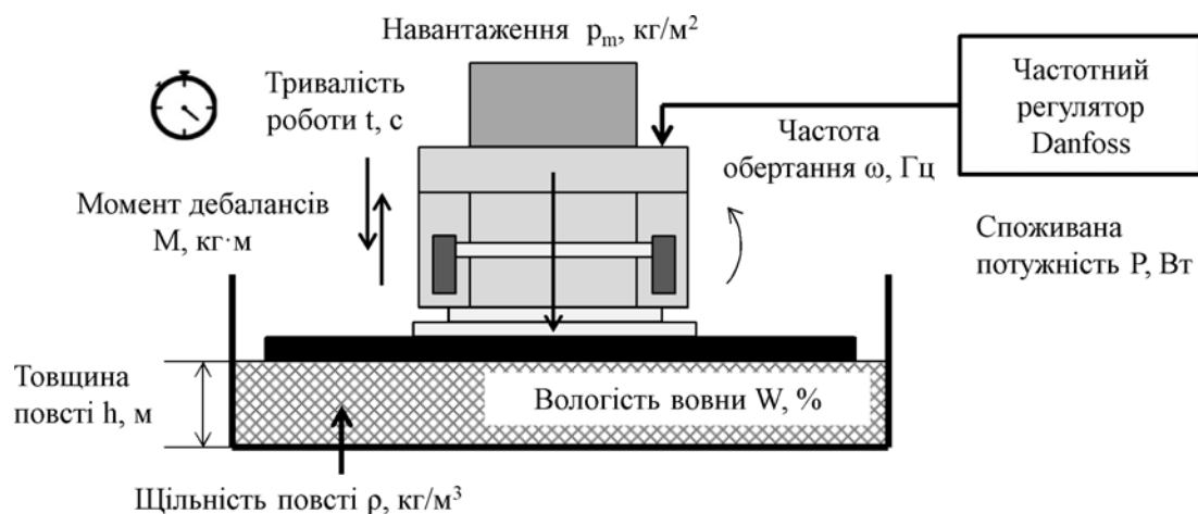
Рисунок 3 – Технологічна схема стенду для експериментальних досліджень
